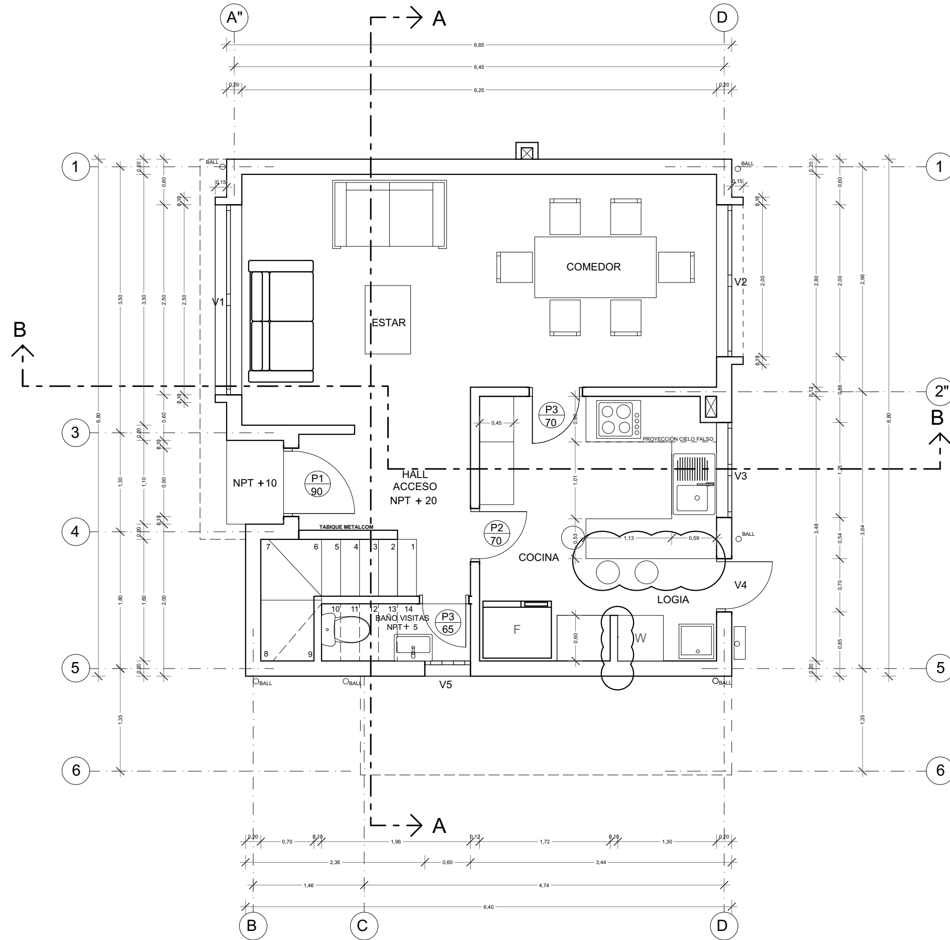
PLANTA NIVEL 1 CASA TIPO A esc: 1:50
