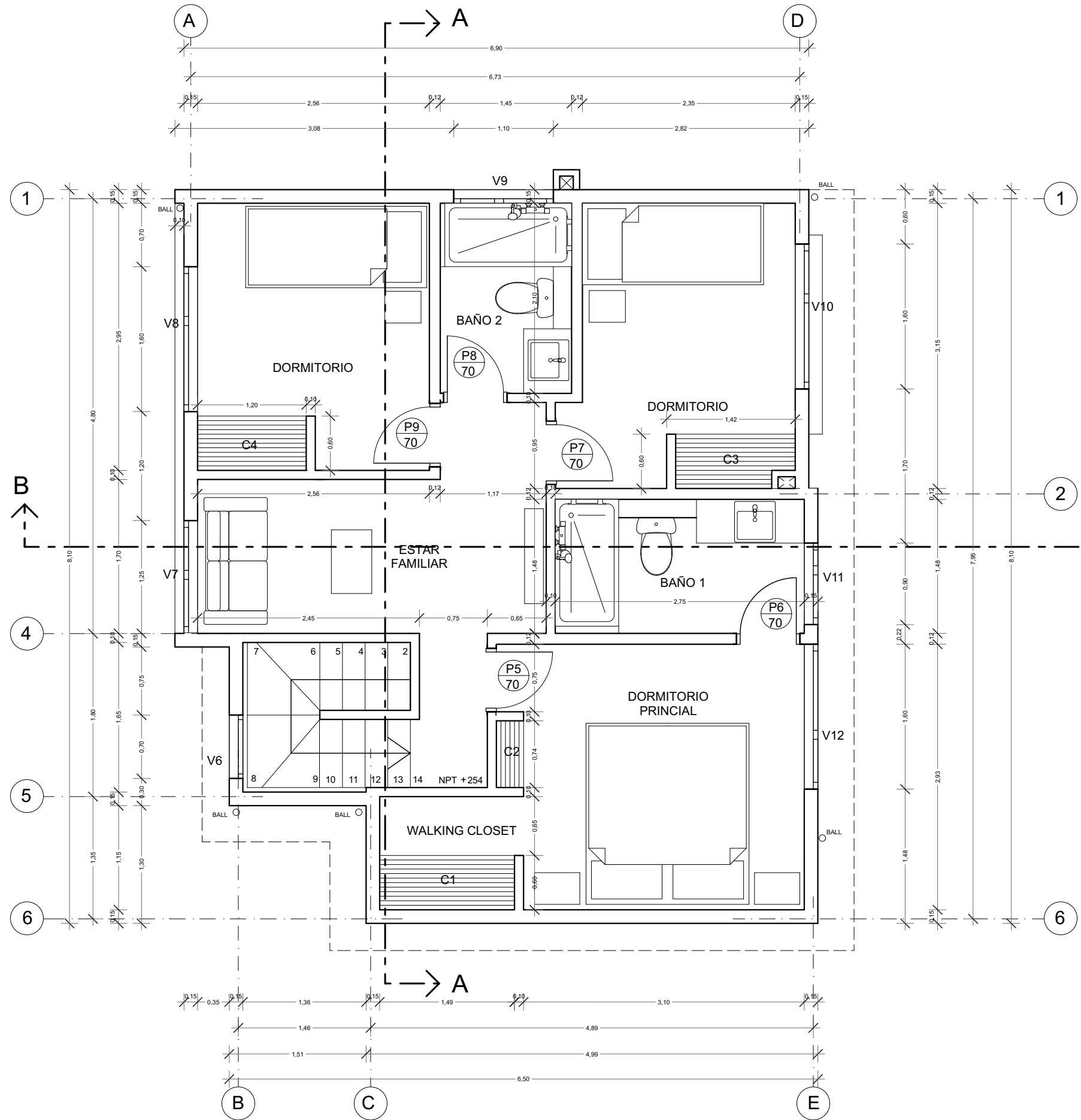
PLANTA NIVEL 2 CASA TIPO A esc:1:50
