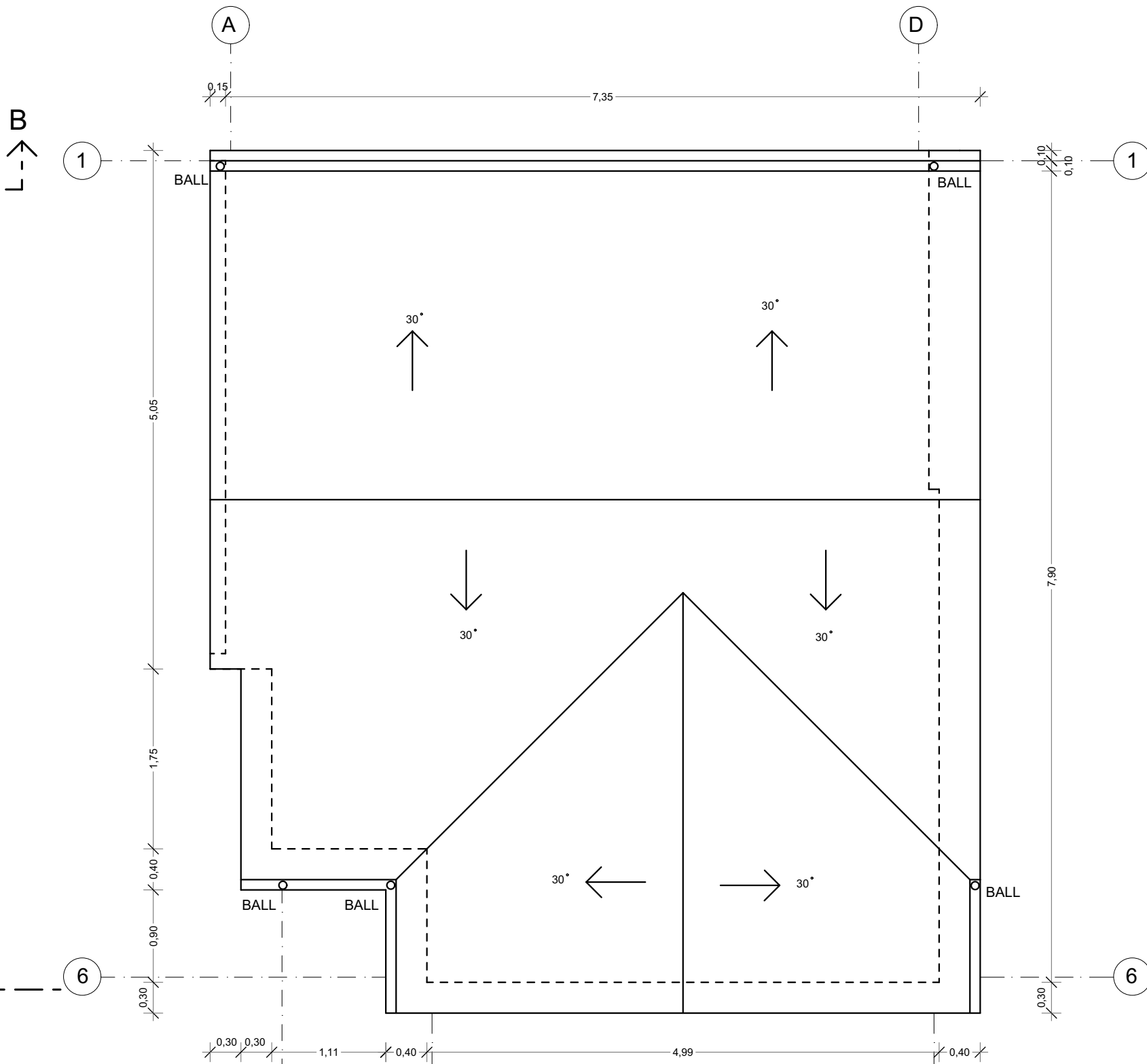
PLANTA TECHUMBRE CASA TIPO A esc:1:50
